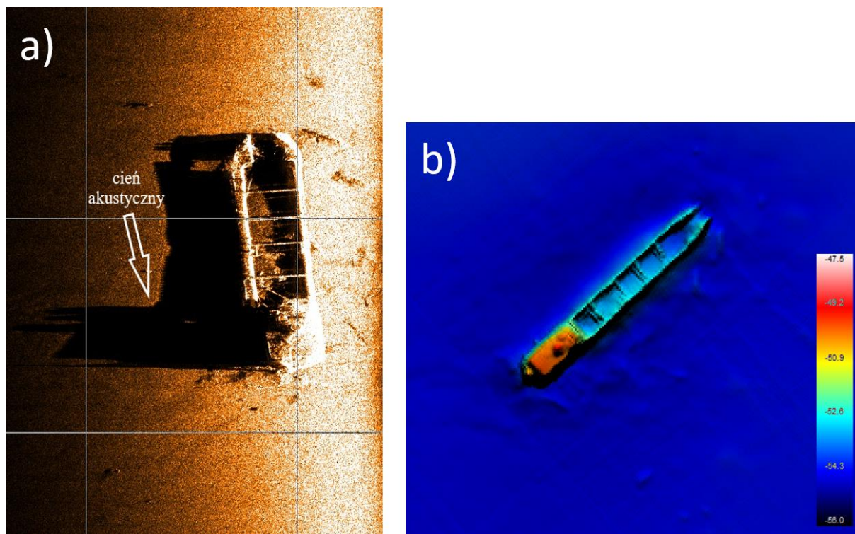
Rys.1. Przykładowe dane zarejestrowane nad wrakiem za pomocą sonaru bocznego (a) i echosondy wielowiązkowej (b) podczas rejsu na statku r/v Oceanograf. Dane zgromadzone, opracowane i zwizualizowane w oprogramowaniu Qinsky.
