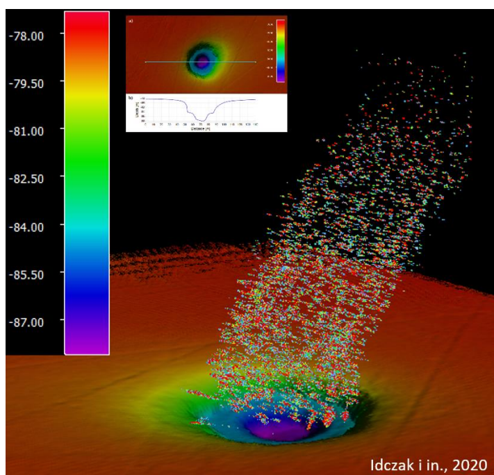
Rys.2. Dane prezentujące pokmark gazowy z widocznymi pęcherzykami gazu uwalnianymi do kolumny wody. Dane zarejestrowane za pomocą echosondy wielowiązkowej ze statku r/v Oceanograf. Zaawansowana obróbka danych z wykorzystaniem programów: Qinsky, Qimera oraz Fledermaus.
